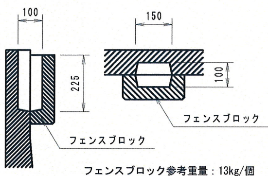
フェンス穴寸法
