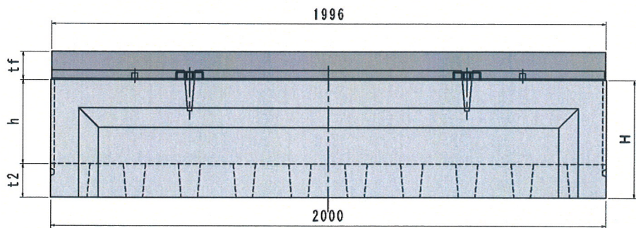
側面図
