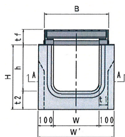
規格寸法及び参考重量
