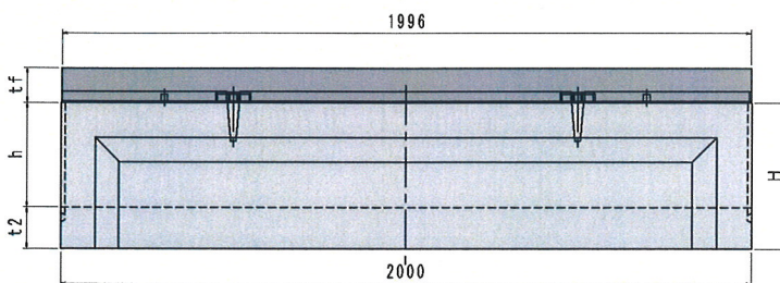
側面図
