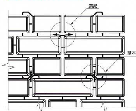
基本 拡大図
