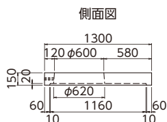
■ 頂版 (H=150, 471kg)
