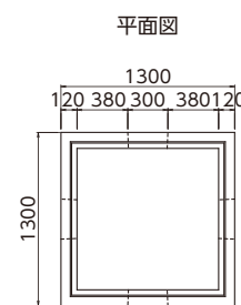
■ 中間部 (H=1000, 1415kg)
