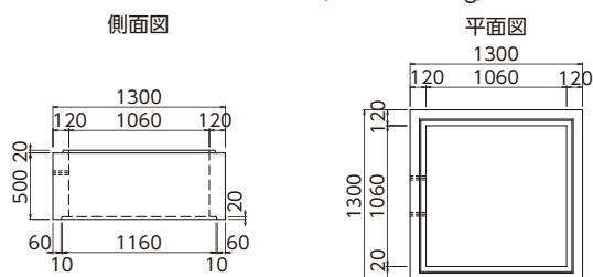
■ 高さ調整中間部 (H=500, 708kg)
