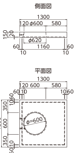
■ 頂版 (H=150, 471kg)
