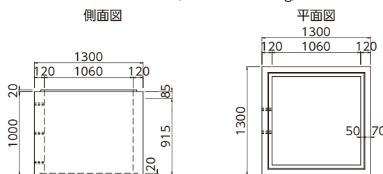
■ 中間部 (H=1000, 1415kg)
