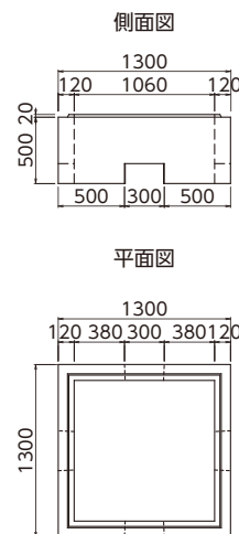
■ 底板兼用穴明き中間部 (H=500, 665kg)
