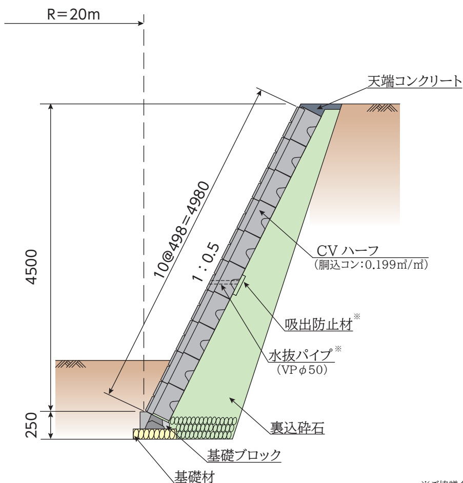
標準断面図
