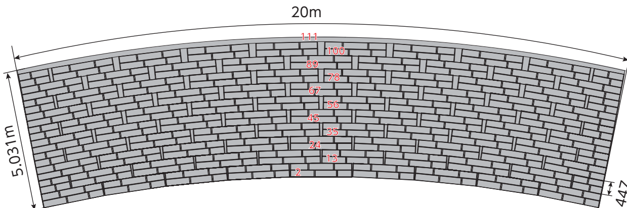
展開図
