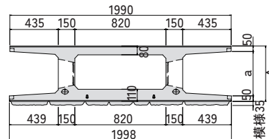
C-C 矢視図
