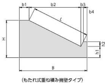
(もたれ式重ね積み擁壁タイプ)
